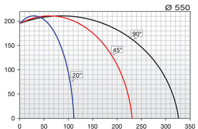
Σχεδιαγράμματα κοπής
